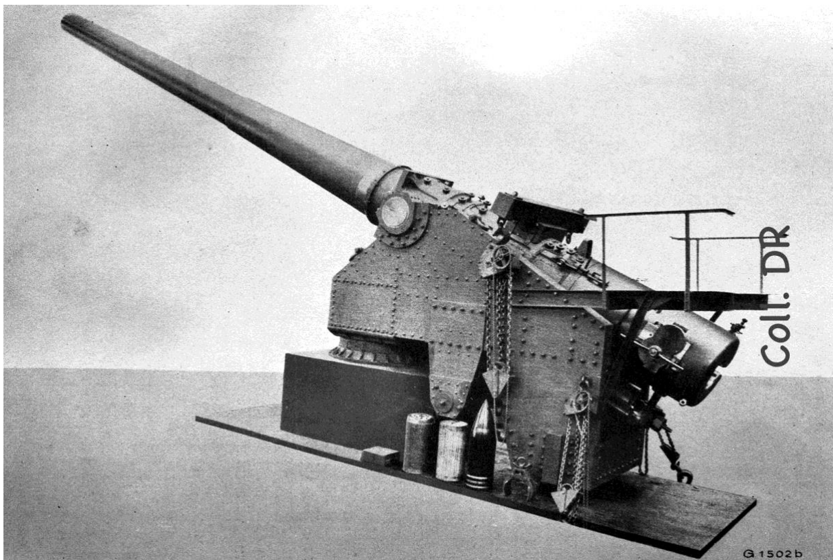
Canon de 38 cm sur affût de polygone, comme celui installé début 1915 devant Verdun.
